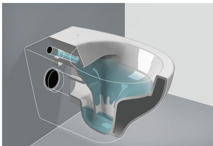
Sistema rimAWAY RimAWAY system Sistema rimAWAY Système rimAWAY
