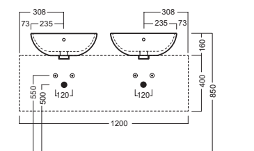
SLIDING wood system_taglio 4 doppio - cut 4 double
